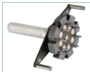
▲ SAMOCENTRUJĄCY UCHWYT MAGNETYCZNY DO ZMIANY SZCZEK
